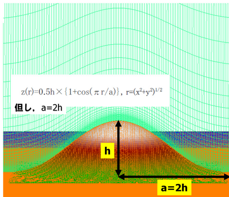
図13 地形近傍の計算格子図
