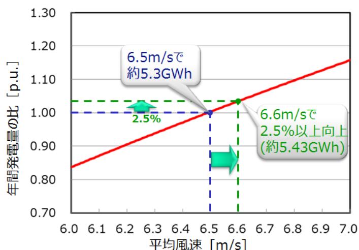
図1 平均風速と年間発電量の関係（標準的な2MW機）
