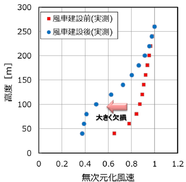
図4 風車建設前後での風況計測結果例
