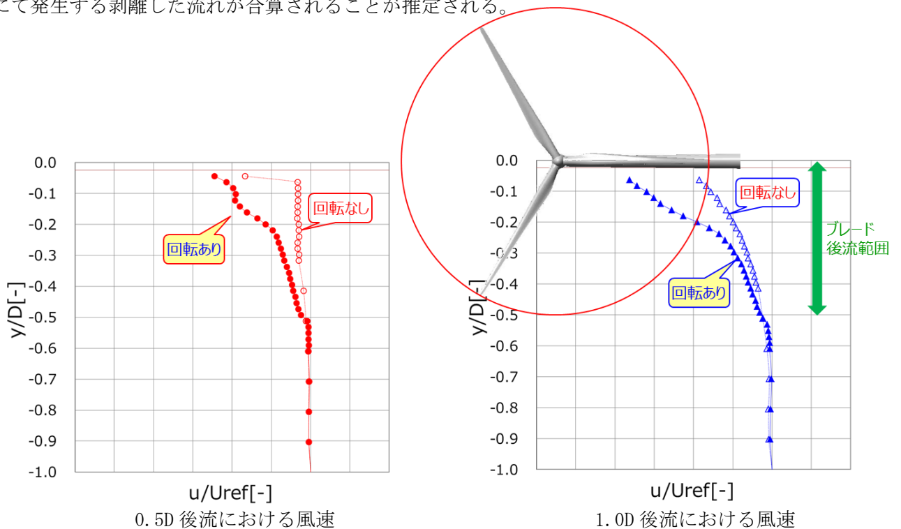
図 11 風車回転時と静止時の後流における風速欠損の比較
