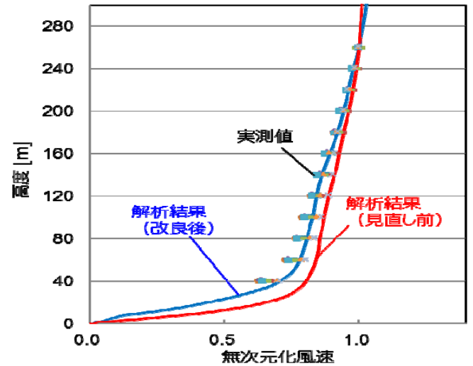
図3 風況解析と風況実測の比較結果
