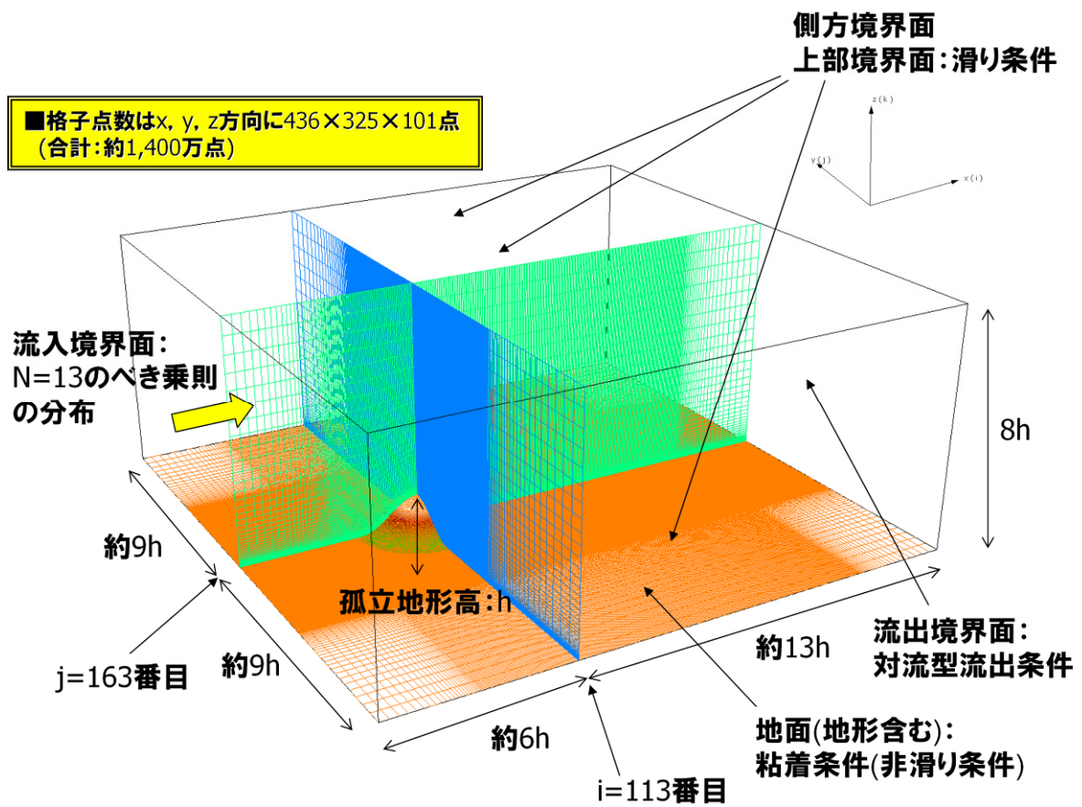
図12 計算領域と境界条件
