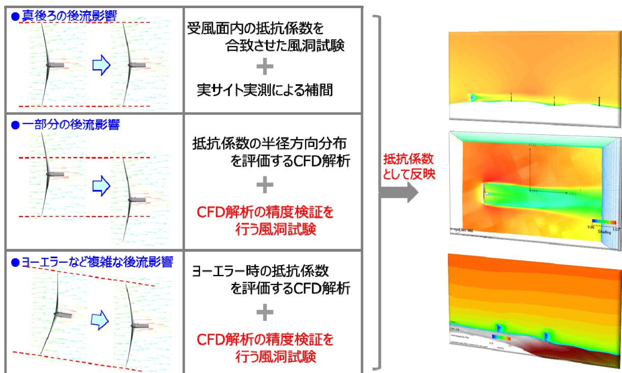
図15 風車後流影響の風況解析への組み込み
