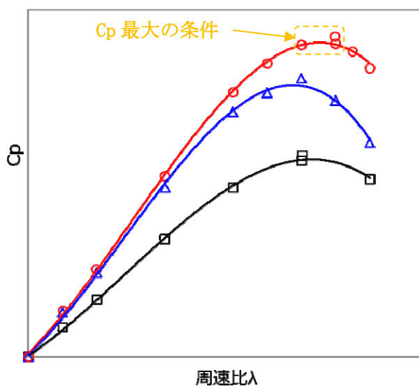
図9 風車模型ブレードにおける周速比 \lambda と圧力係数 C_p の関係
