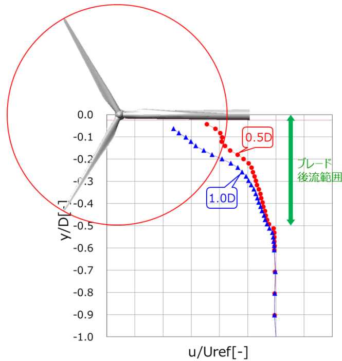
図 10 風車後流の欠損量評価結果
