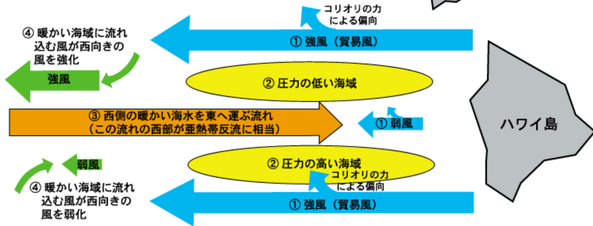
図6 ハワイ諸島西側において島陰が発達するメカニズム
