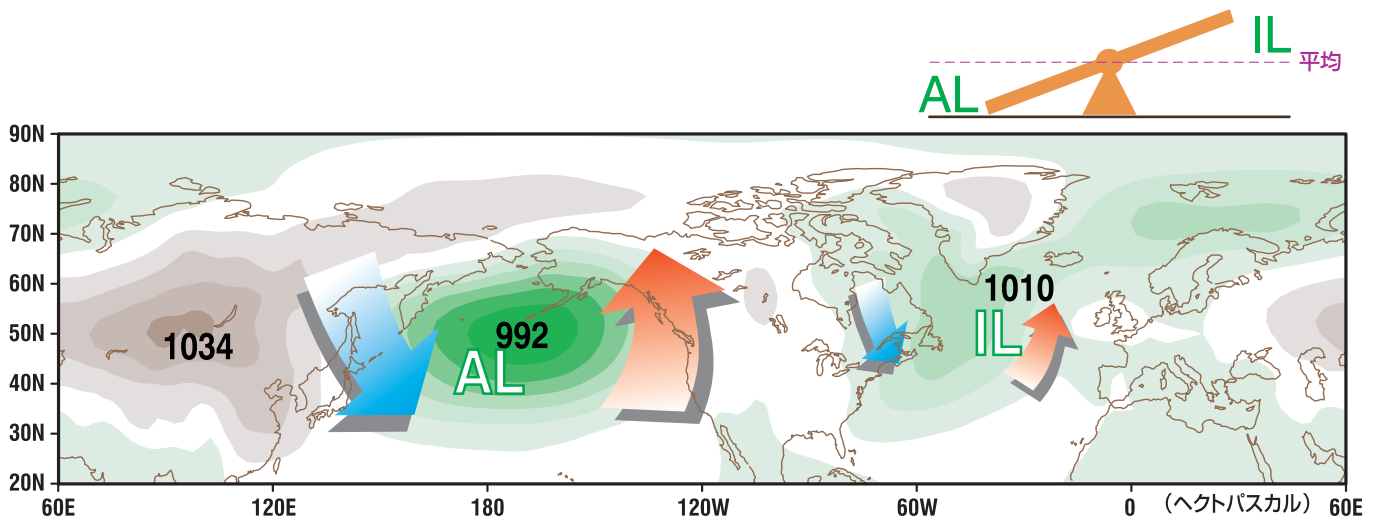
図1a. アリューシャン低気圧(AL)の勢力が強い年の典型的な海面気圧の分布図 (2月10日~3月12日の平均)
