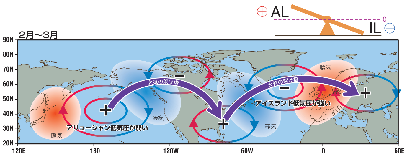
図1c. 「大気の架け橋」の形成過程模式図
