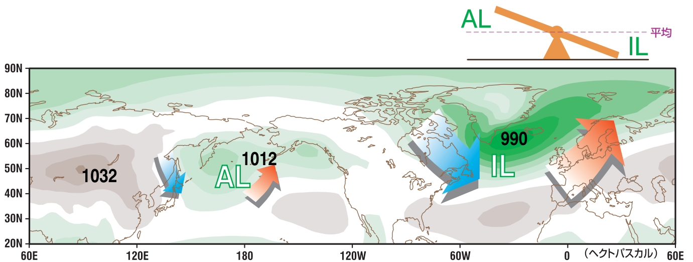
図1b. アイスランド低気圧(IL)の勢力が強い年の典型的な海面気圧の分布図 (2月10日~3月12日の平均)
