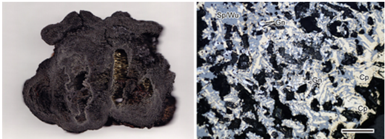
図3 採取した人工熱水噴出孔チムニー
