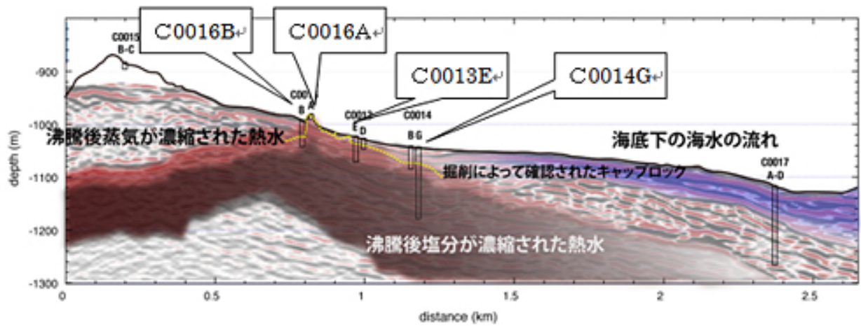
図2 IODP第331次研究航海で設置した人工熱水噴出孔（4地点）の位置関係
