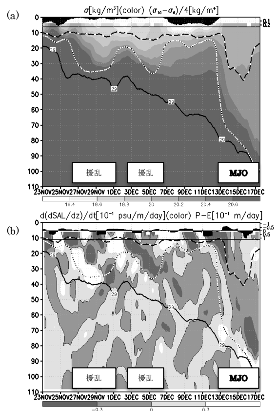
図1: 研究船「みらい」のCTD(3時間毎)による深度時間断面図(a)密度( \text{kg/m}^3 )、(b)塩分鉛直傾度の時間変化( \times 10^1 \text{psu/m/day} )。 (a)の上部は、水深6-10mの密度鉛直傾度( \text{kg/m}^4 )、表層淡水化指標、右軸、(b)の上部は、淡水流量( \times 10^1 \text{m/day} 、降水と蒸発量の差、右軸で海洋に流入する成分を正)を示す。破線と点線は、水深10mを基準に 0.2^\circ\text{C} 相当の密度差で定義された混合層、水温差 0.2^\circ\text{C} で定義された等温層。太い実線は、 29^\circ\text{C} の等温線で示されている。全ての変数は、潮汐変動を除くために24時間の移動平均をかけた。
