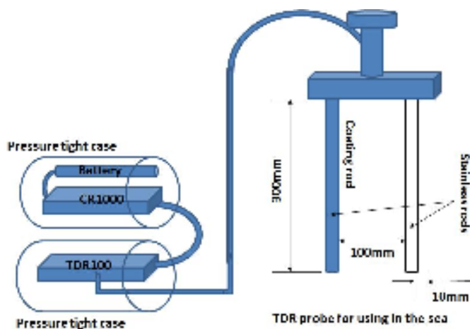
図1 海底土壌における測定装置
