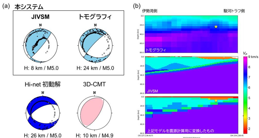
図 2-1-②-2 (a) 地震 A の発震機構解。左上は JIVSM、右上はトモグラフィモデルを用いて本システムで求めた初動解（水色）。左下は 1D 構造モデルに基づく防災科研 Hi-net による初動解（青色）。右下は 3D-CMT 解析結果 7) （桃色）。各発震機構解下部には、それぞれの解析により得られた震源（セントロイド）深さ及びマグニチュードを表す。(b) 計算に用いた P 波速度構造の鉛直断面図。断面線の位置は、図 2-1-②-1 に示す。断面図中の星印は、それぞれのモデルで求めた震源の概略位置を表す。
