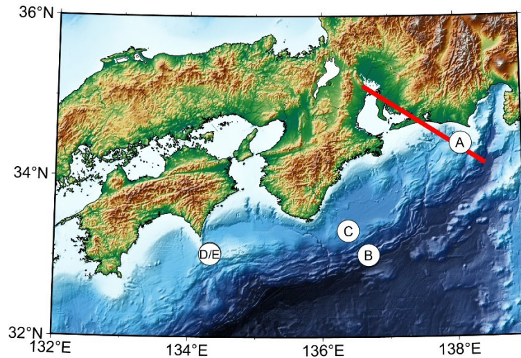
図 2-1-②-1 初動解の評価対象とした地震の震源分布。図中の A～E は表 2-1-②-1 に対応する。また、赤線は図 2-1-②-2 の断面線の位置を表す。
