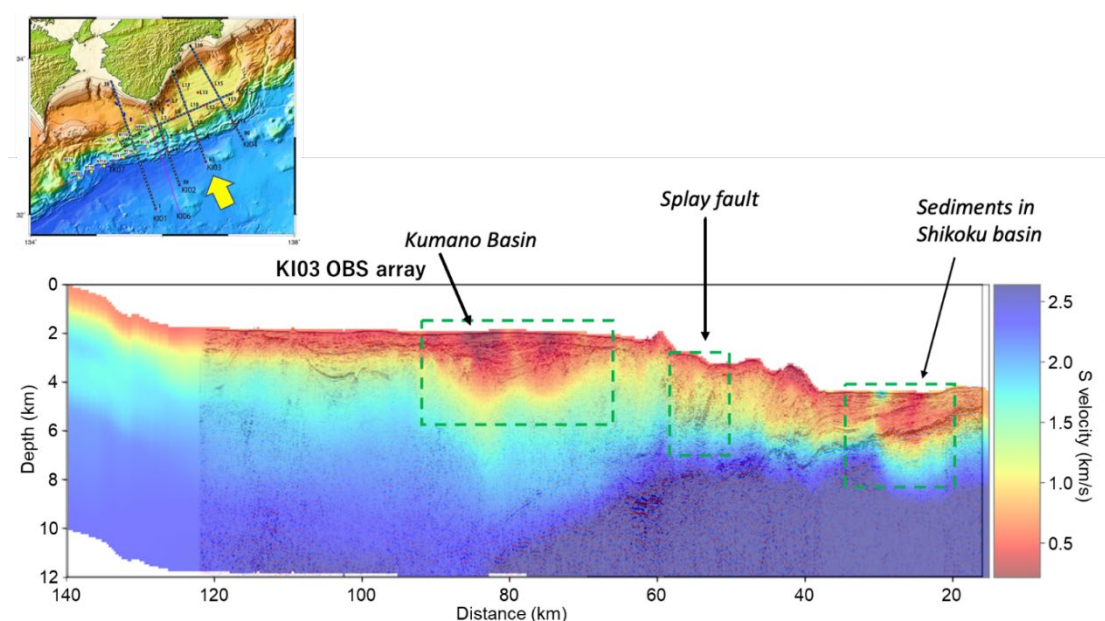
図1 紀伊半島沖熊野灘の測線（地図の矢印）下のS波速度構造。測線上に5 km 間隔で設置した海底地震計で観測されたノイズデータから表面波を抽出し、逆解析によりS波速度モデルを構築した。同海域で取得した反射法地震探査データで堆積層が厚くイメージされている熊野海盆で低S波速度領域が厚くなるなど、反射法探査の解析結果と整合的なS波速度構造モデルである。
