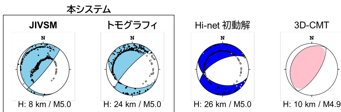
図2 2011年8月12日に遠州灘で発生した地震の発震機構解。水色で示した2つの解は開発中のシステムによる初動解であり、左側は全国1次地下構造モデル（JIVSM）、右側は地震波走時トモグラフィ（Matsubara et al., 2019）に基づく3D構造を用いた結果である。青色及び桃色で示した解は、それぞれ、1D構造を用いた初動解、3D構造モデルを用いたセントロイドモーメントテンソル（CMT）解（Takemura et al., 2021）を示す。各解の下部にそれぞれの方法で求めた震源深さとマグニチュードを示す。沈み込むフィリピン海プレートを明瞭にモデル化したJIVSMに基づく3D構造モデルを用いることによって、CMT解に比較的類似した発震機構解が得られたことが分かる。
