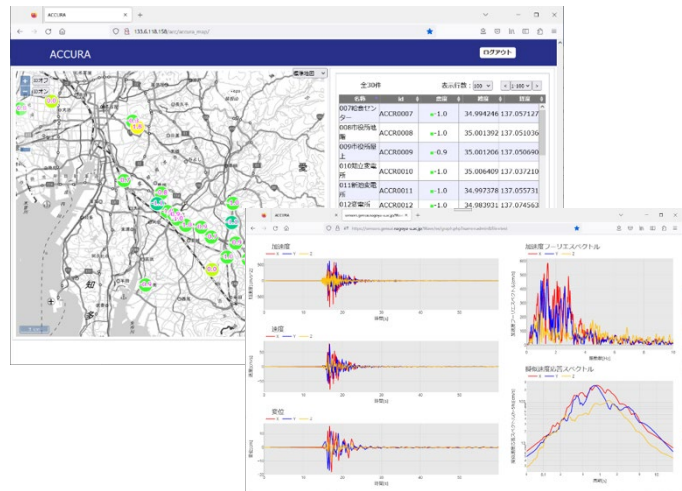
図9 既存の震度計配置を補間する連続モニタリングシステムの開発
