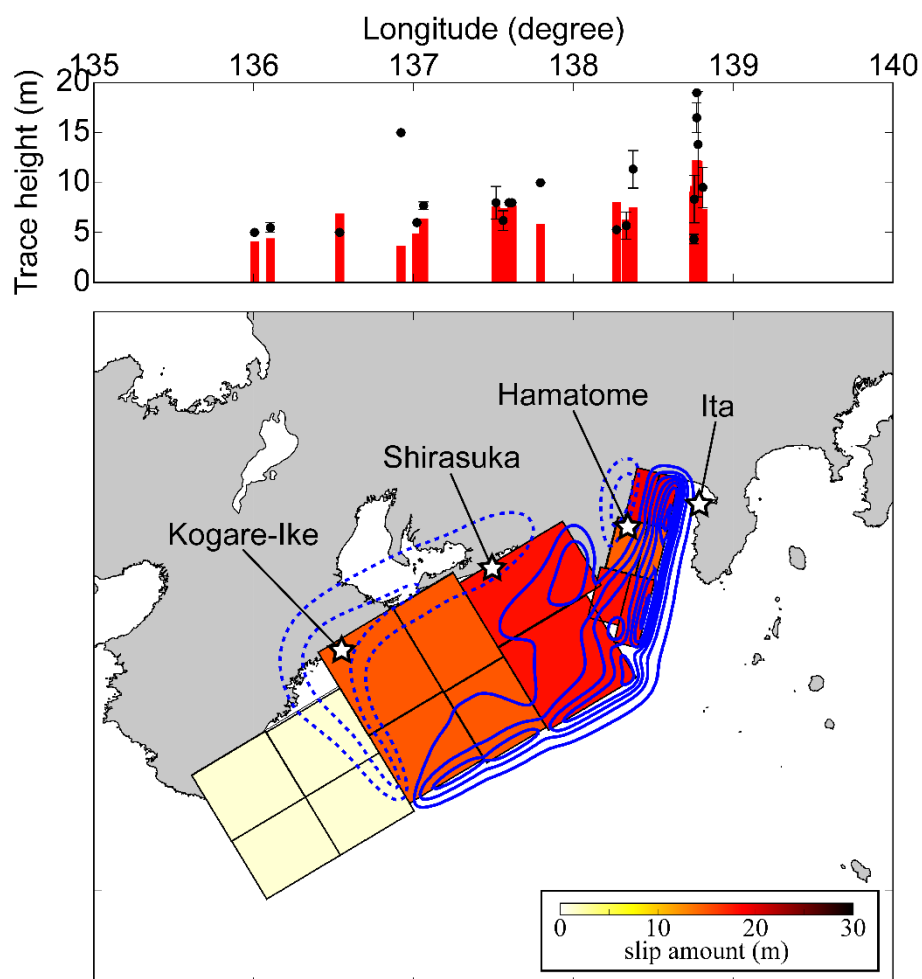
図5 津波痕跡高と津波堆積物調査地の浜提高さに基づいた 1498 年明応東海地震の津波波源モデル。星印は津波堆積物調査を実施した調査地（三重県南伊勢町こがれ池・静岡県湖西市白須賀・静岡県焼津市浜当目・静岡県沼津市井田）の位置を示す。
