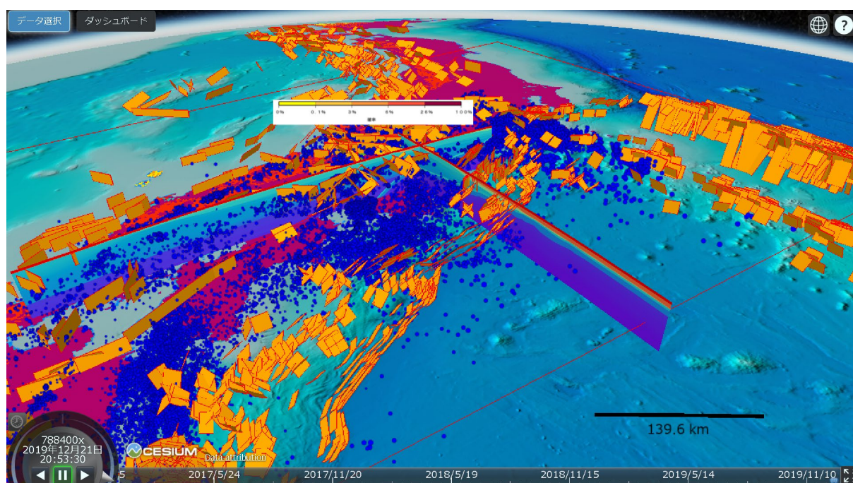
図 16 地殻活動監視ダッシュボードの表示例。サブ課題 1 から提供された震源分布、サブ課題 2 から提供された今後 30 年間に震度 5 弱以上の揺れに見舞われる確率、既存の海陸活断層分布、地殻構造を比較して表示した。
