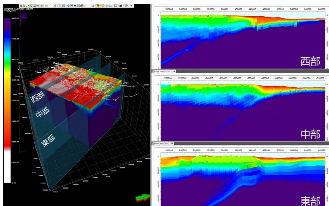
図1 令和5年度に構築したマルチパラメータ3D構造モデル（左）について、南海トラフ域の西部、中部、東部の3箇所を北東―南西方向に切った断面のP波速度構造（右）。入力した構造情報に基づく沈み込みの東西変化が反映されているが、西部断面（右上）では、各種モデルの統合による不連続が認められる。
