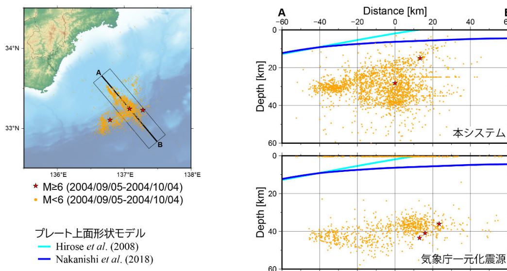
図2 紀伊半島南東沖の震源分布。2004年9月5日から30日間に発生したマグニチュード6以上の地震を赤星印で、それ以外の地震を橙点で示した。右上に3D構造モデルを用いて再決定した震源カタログ、右下に気象庁一元化震源情報の鉛直断面図を示す。断面線の位置は左地図に示す。3D構造モデルを用いることにより、震源の深さが有意に浅くなったことが分かる。
