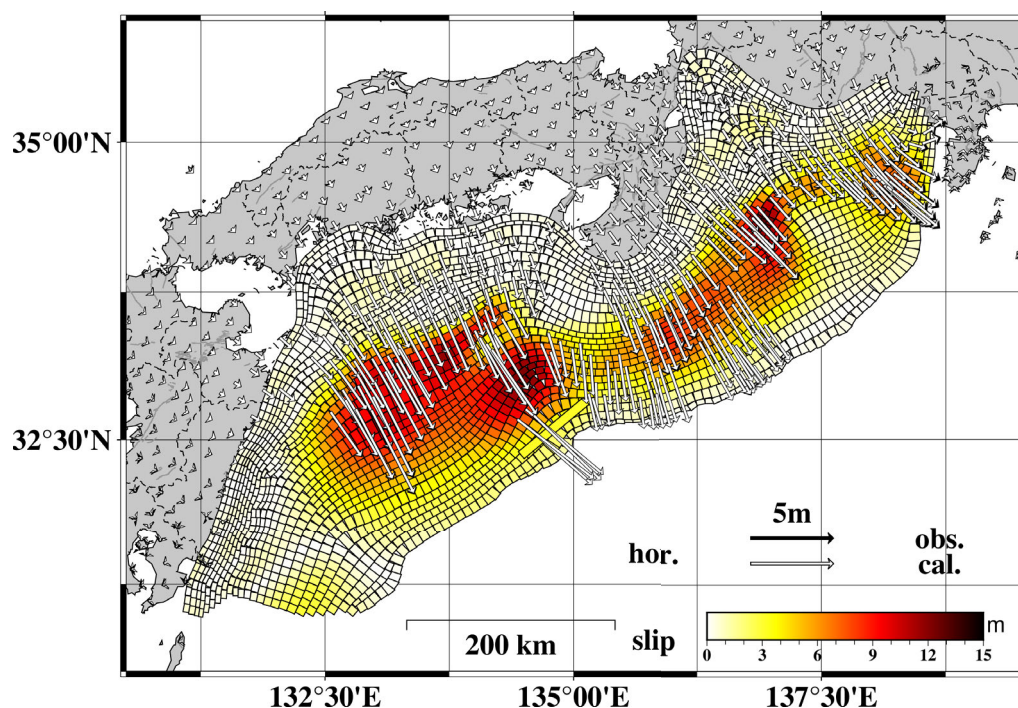
図3 プレート境界におけるすべり分布および同時推定された分岐断層のすべり量。矢印は各観測点における水平変位場を示す。推定には用いていないが、DONET において期待される水平変位場も参考のために併記した。
