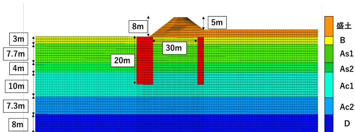
図 2-8-①-9 ローカルモデルの有限要素メッシュ（堤防周辺の拡大図）
