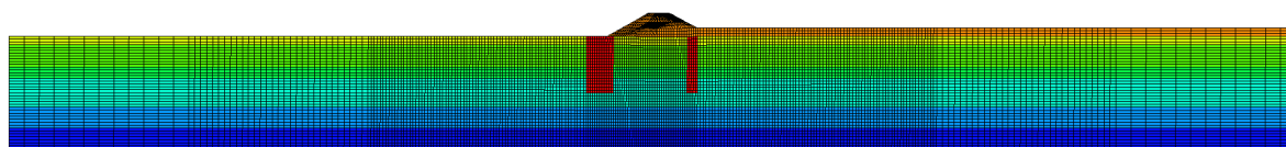
図 2-8-①-8 ローカルモデルの有限要素メッシュ（全体図）
