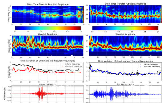
図12 建物被災度判定に向けたウェーブレット変換による建物固有振動数変化のモニタリング
