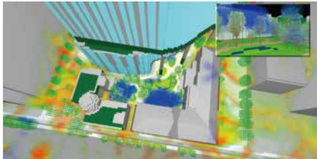
「丸の内パークビル」の樹木がもたらす低温暖化現象のシミュレーション（MSSG モデル） 国立研究開発法人海洋研究開発機構／株式会社三菱地所設計／株式会社竹中工務店
