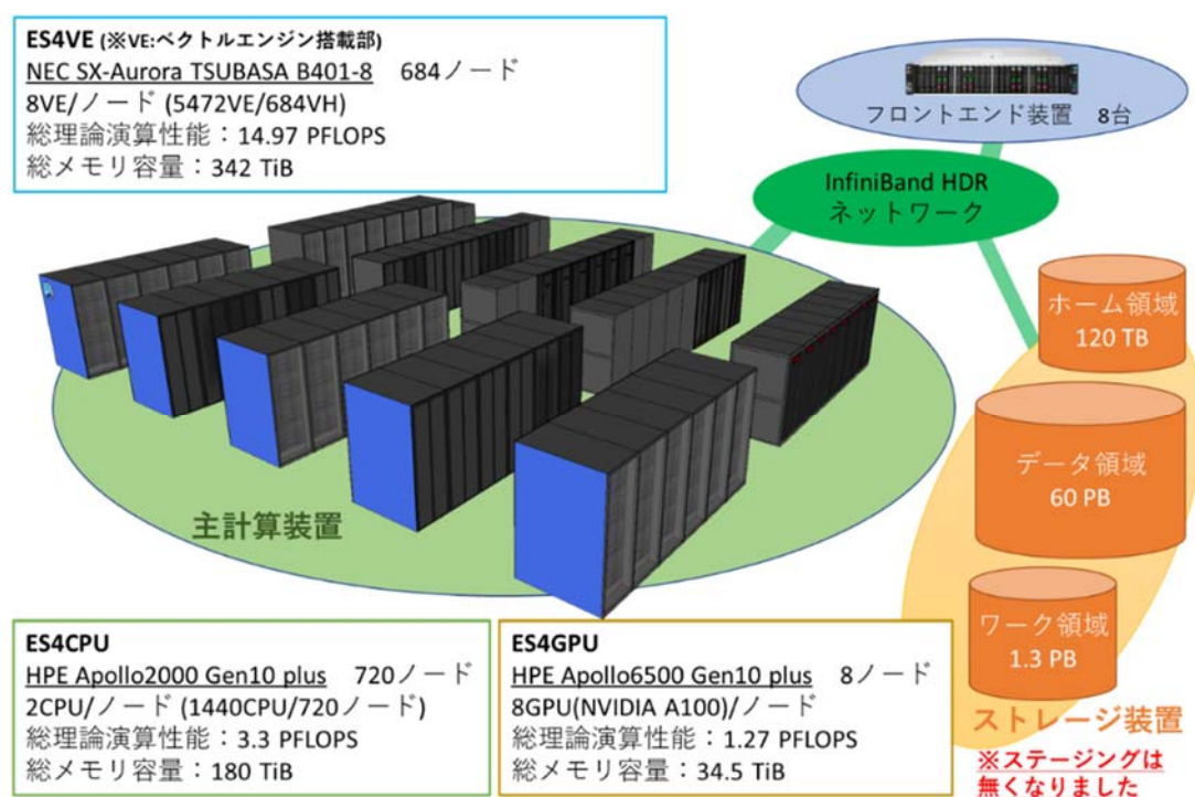
ES4のシステム概念図
