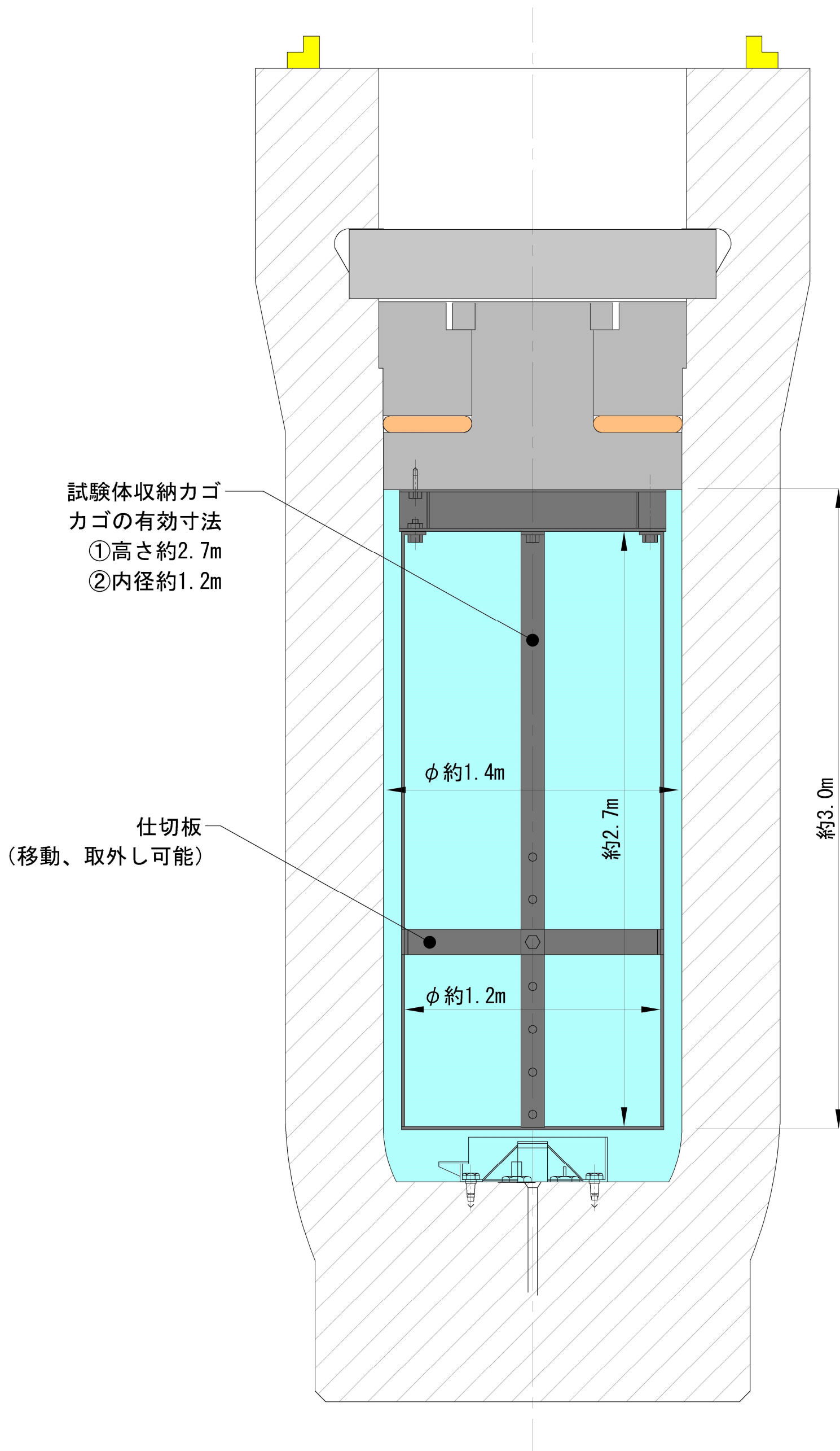
設備の概要(断面図)
