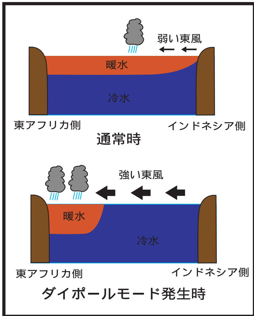
ダイポールモード現象
