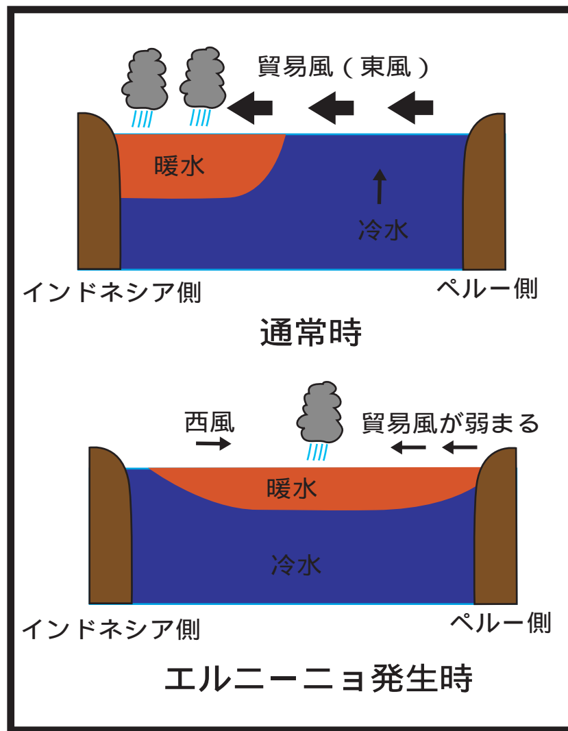
エル・ニーニョ現象
