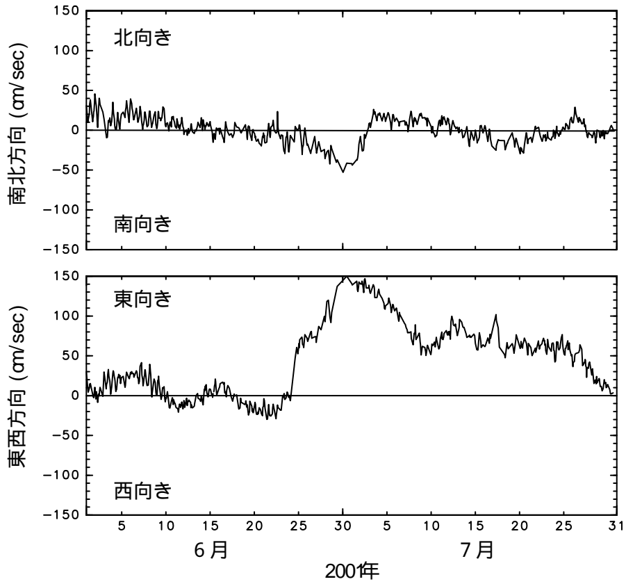
赤道上、東経 156度の深度 10 mの流速
