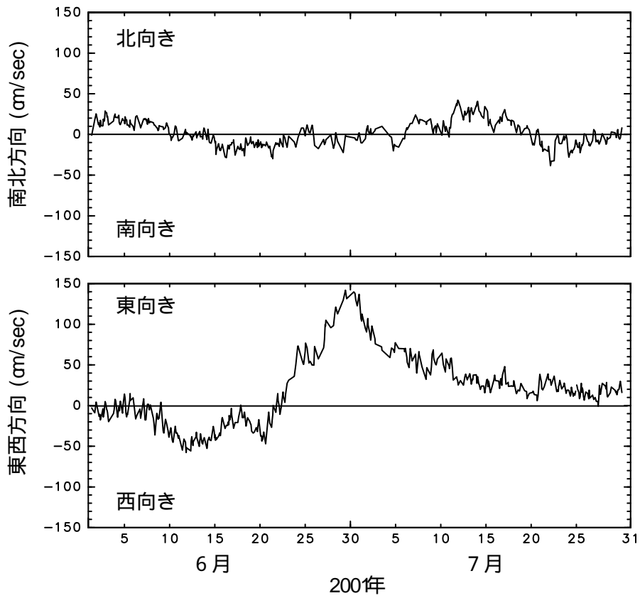
赤道上、東経 14度の深度 10 mの流速
