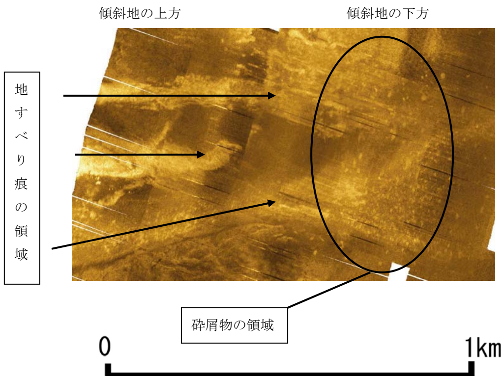
図 2-2 地すべり痕と砕屑物によると思われる強反射の領域
