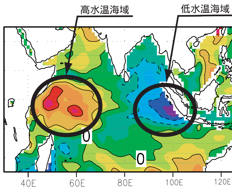
モデルにより再現された ダイポールモード現象
