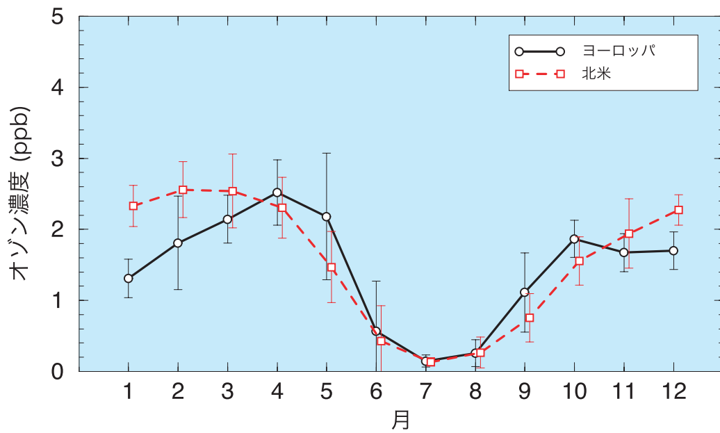
図2：日本（八方）に対するヨーロッパと北米からのオゾン影響の季節変化。 □ (1996年の月平均値) □ ヨーロッパからの影響は4月に最大、北米からの影響は2，3月にピークとなる。
