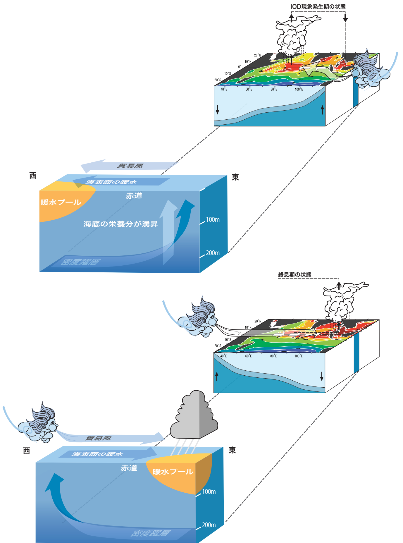
図2：IOD現象発生期（上図）及び終息期（下図）の大気海洋相互作用（風、海洋内部、降雨）の模式図
