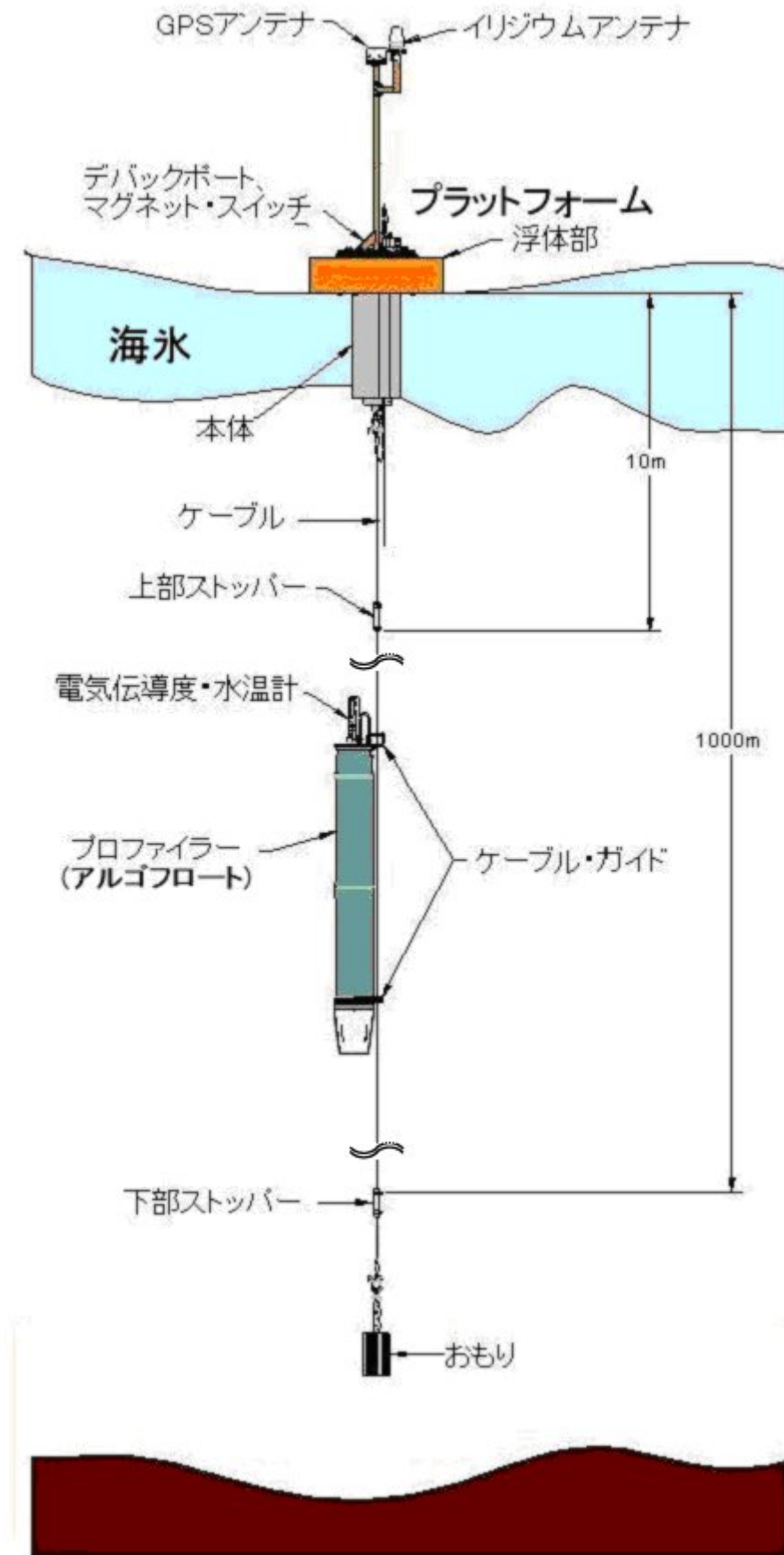
図1 POPS (Polar Ocean Profiling System: 氷海用観測システム) の模式図。
