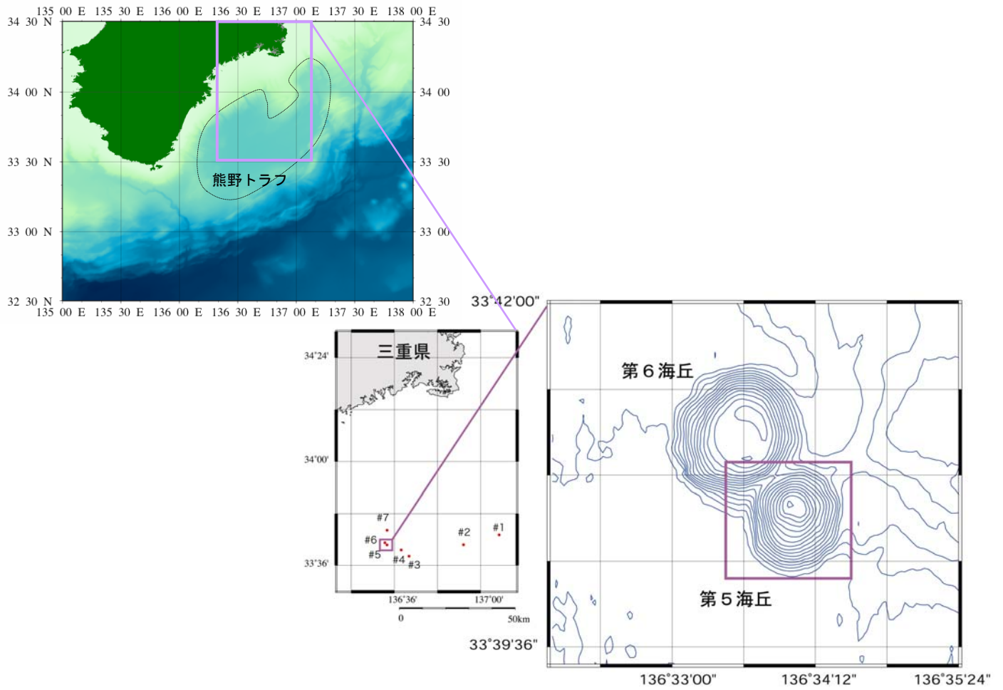
図1 「うらしま」による調査海域図
