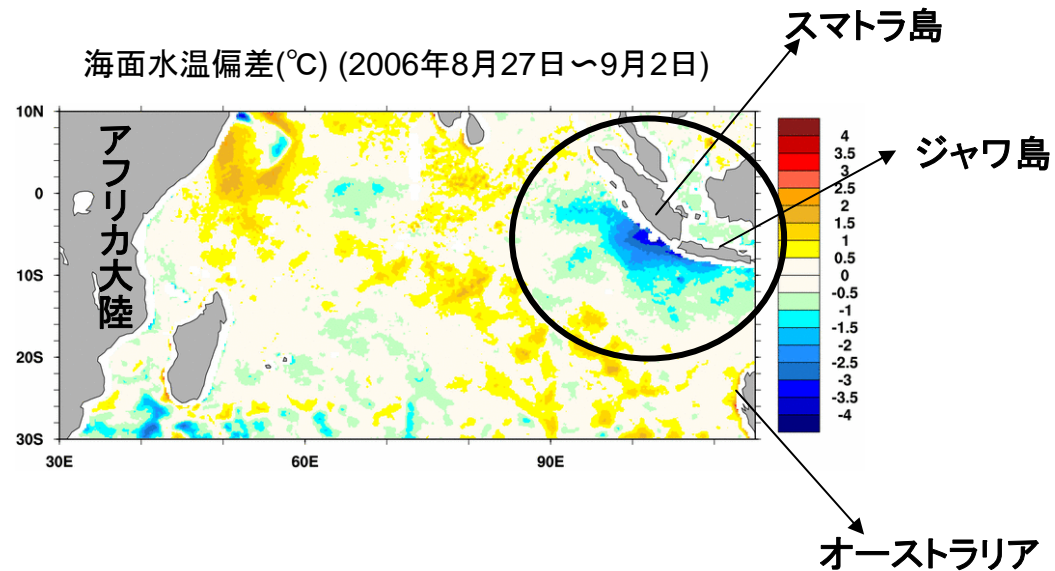
図3:人工衛星から観測された2006年8月現在のインド洋の状態
