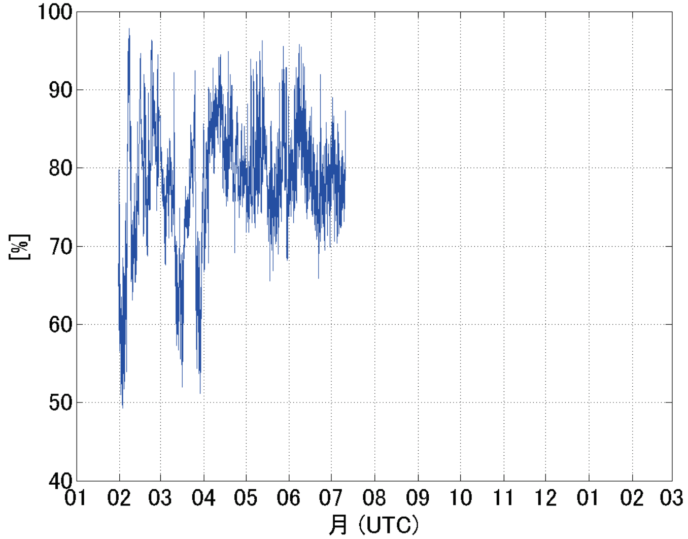
湿度[%] 2012/01/31~13/02/20
