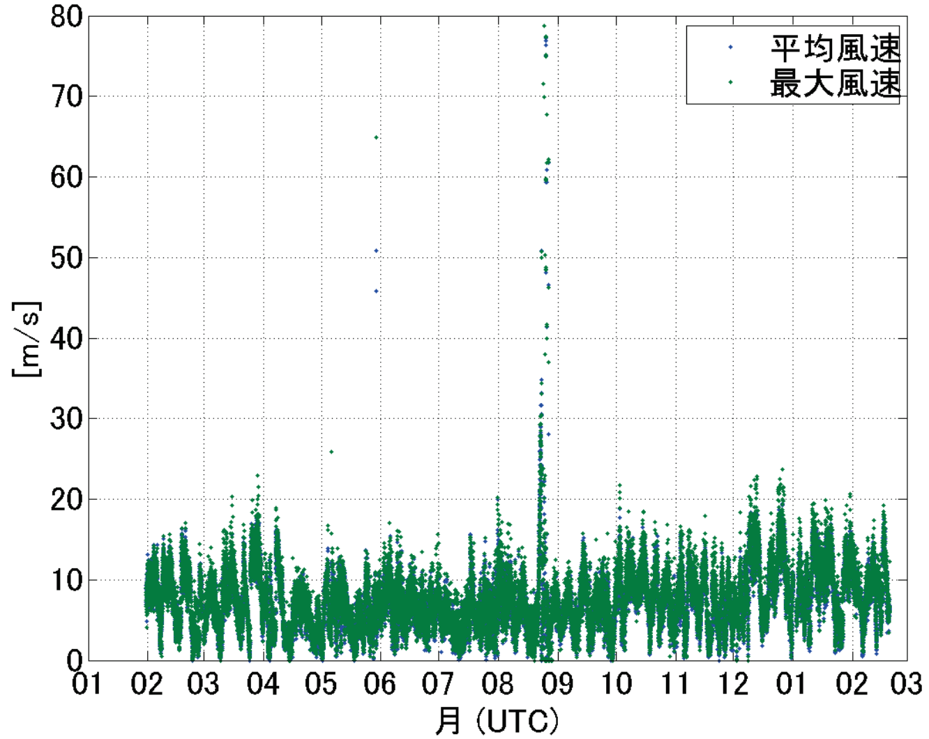
風速[m/s] 2012/01/31~13/02/20
