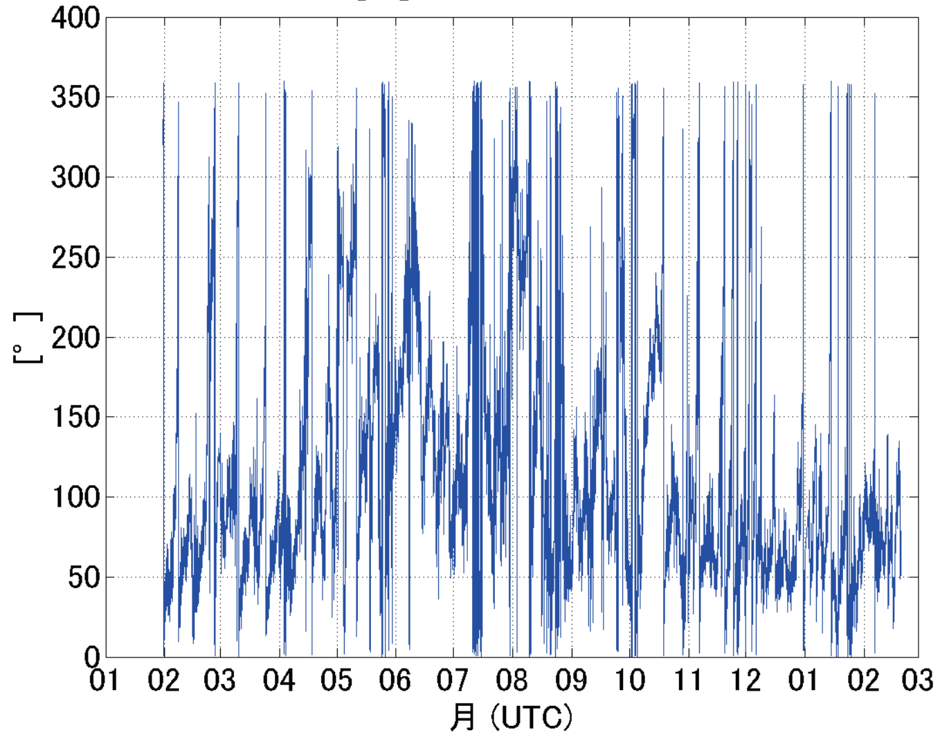
風向[° ] 2012/01/31~13/02/20
