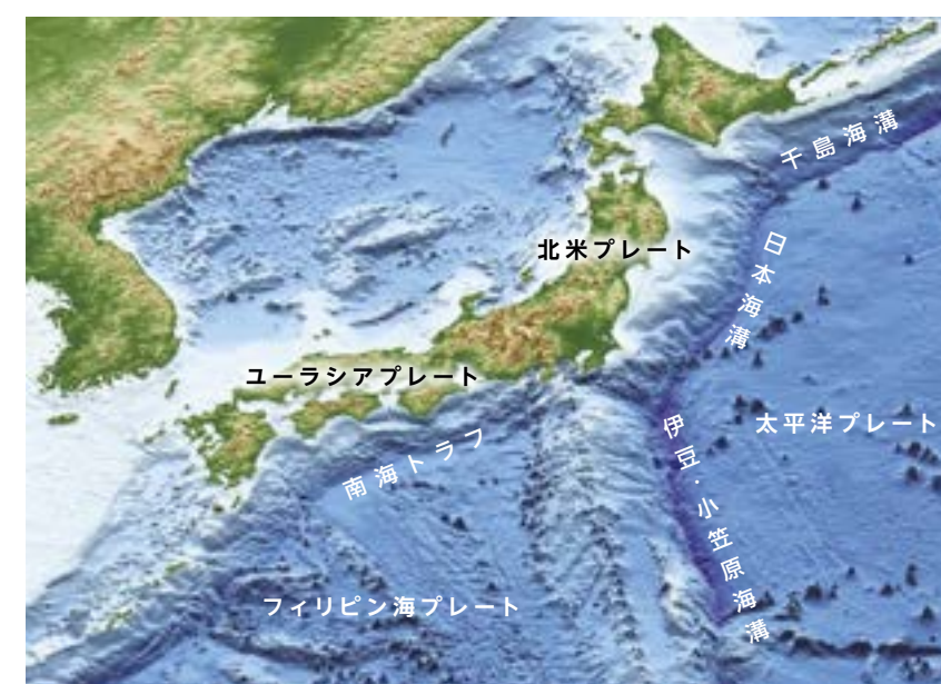
日本周辺のプレート
