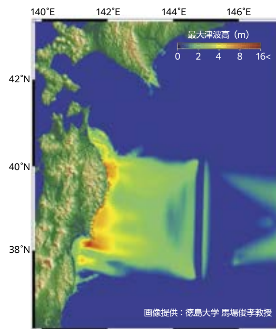
アウターライズ地震による津波高の予測 M8.7のアウターライズ地震が起きた場合
