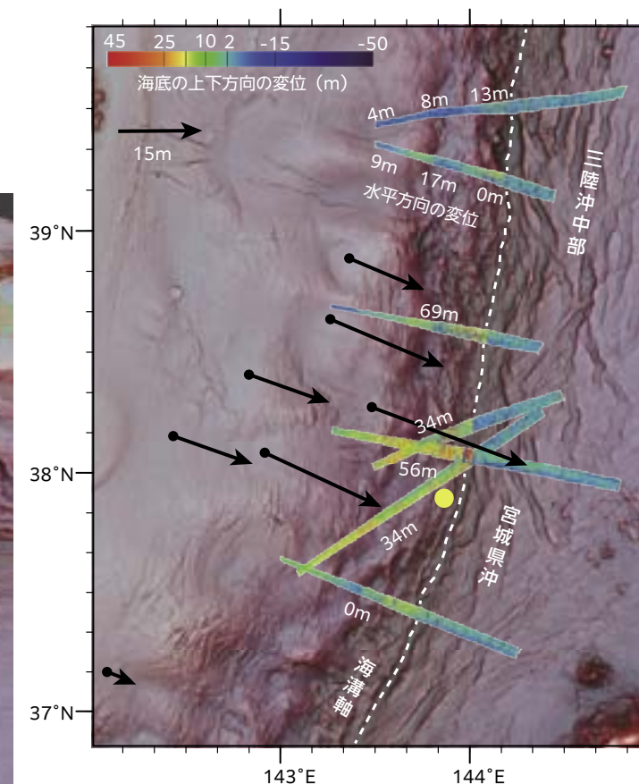
宮城県沖の黄色の点は、東北地方太平洋沖地震調査掘削 (JFAST) の掘削地点 (本誌10~11ページ)。
