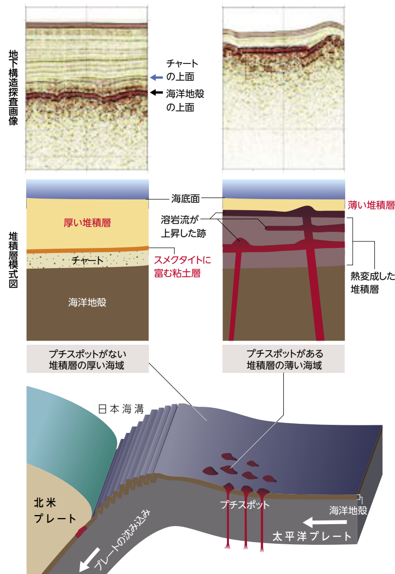
プチスポットと堆積層の厚さ
