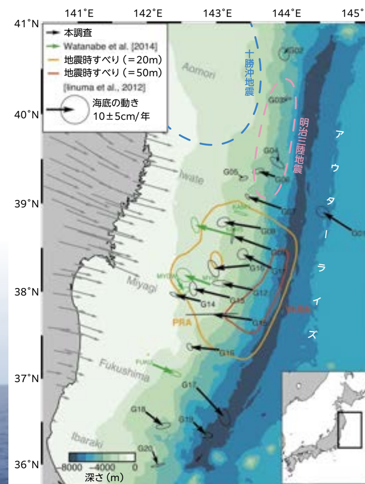
東北沖の海底の動き（2012年9月～2016年5月）
