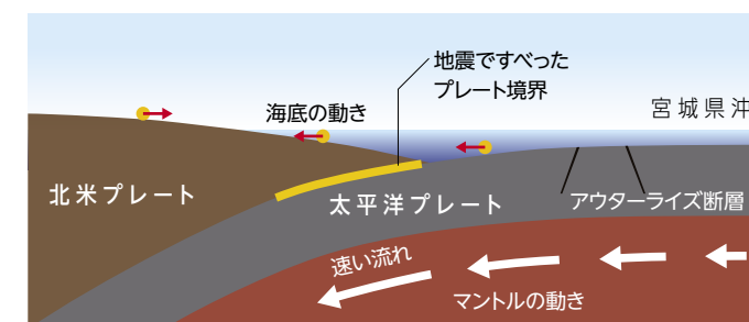
地震後のマントルの動き
