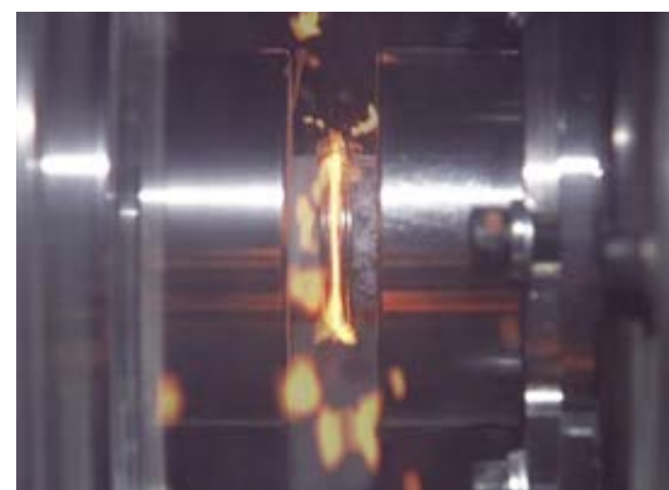
地震時の高速すべり再現実験
