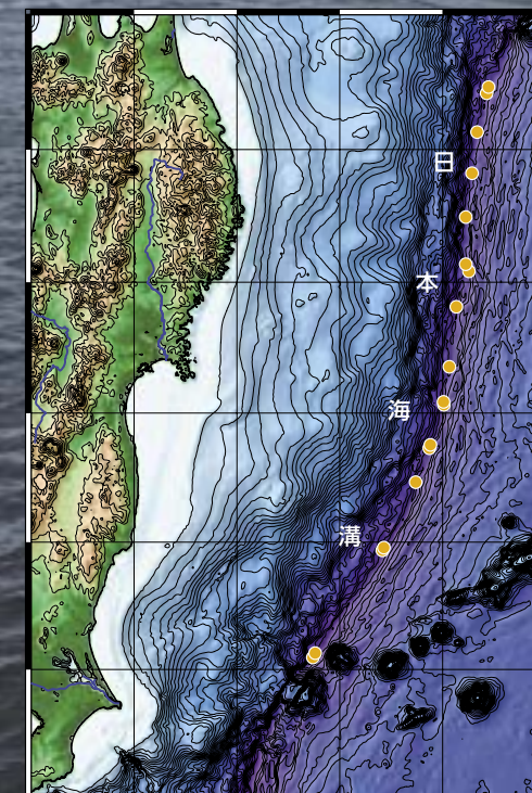
IODP第386次研究航海の掘削地点（黄色）
