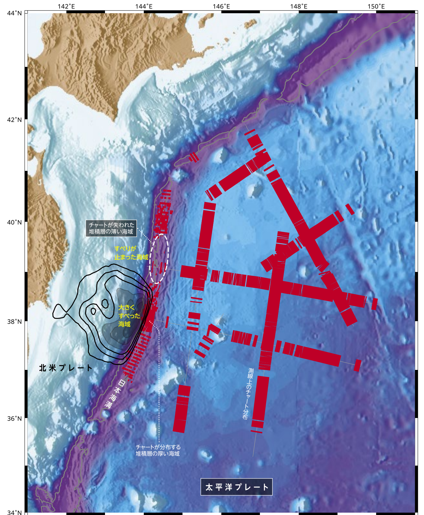
堆積層の厚さに対応するチャート分布 (赤)
