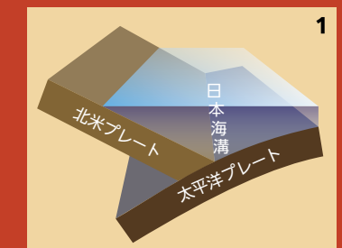
日本海溝のプレート境界で起きる地震の概念的な発生メカニズム
