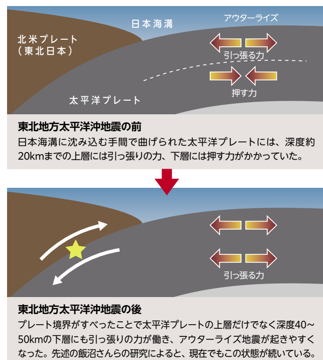
アウターライズ地震が誘発される状態
