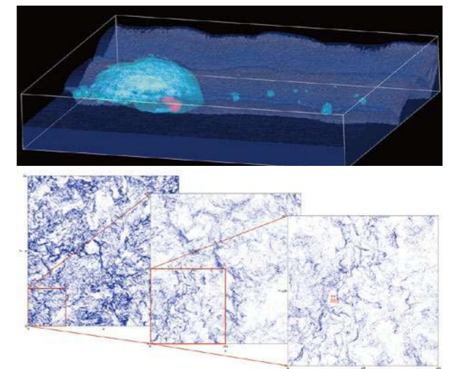
上：大規模粒子体計算で再現する地震現象 下：大規模データ解析が明らかにする雲粒クラスタの階層構造
