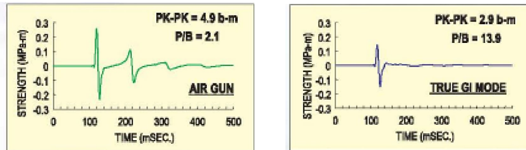
図-3 エアガン波形比較
