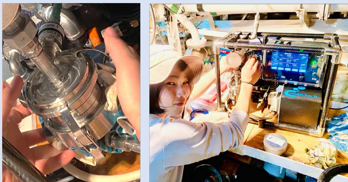
図2（左）半自動マイクロプラスチックサンプラーのフィルターカセット部分。（右）マイクロプラスチックサンプラーのフィルターを交換する調査チーム 関友理恵（ヤマハ発動機）。
